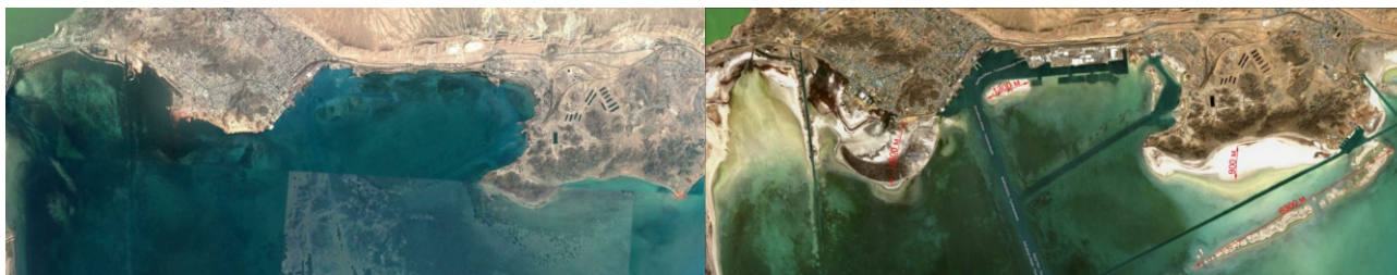
Снимки побережья у г. Туркменбаши в 2004 и 2023 гг. (Источник: https://meteojournal.ru/kaspkom-2023-godu-iz-za-malo-vodya-na-volge-tretij-god-podryad-uroven-kaspijskogo-morya-prodolzhit-ponizhatsya/ )
