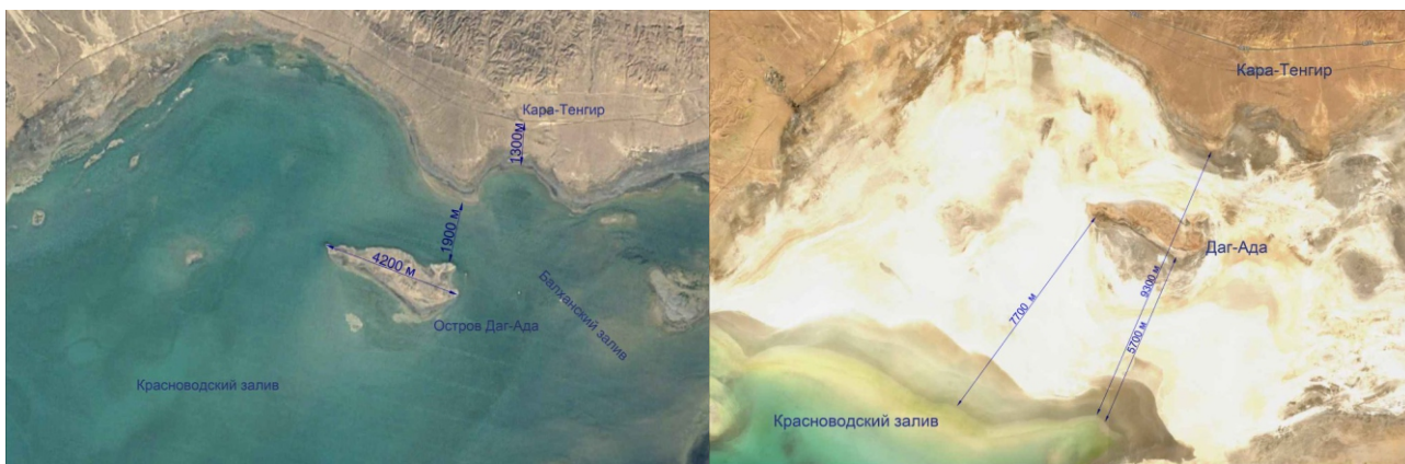
Снимки острова Даг-Ада в 2009 и 2023 гг. (Источник: https://meteojournal.ru/dag-ada-ostrov-kotorogo-net/ )
