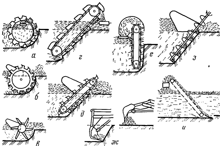
Рис. 9.2. Схемы рабочих органов различных дренажных машин: а — колесный рабочий орган траншейного канавокопателя; б — дисковая фреза; в — скребковое колесо; г — многоковшовый цепной рабочий орган; д — цепной рабочий орган фрезерного типа; е — скребковый цепной рабочий орган; ж — экскаваторный ковш; з — шнековый рабочий орган; и — дренажный плуг.
