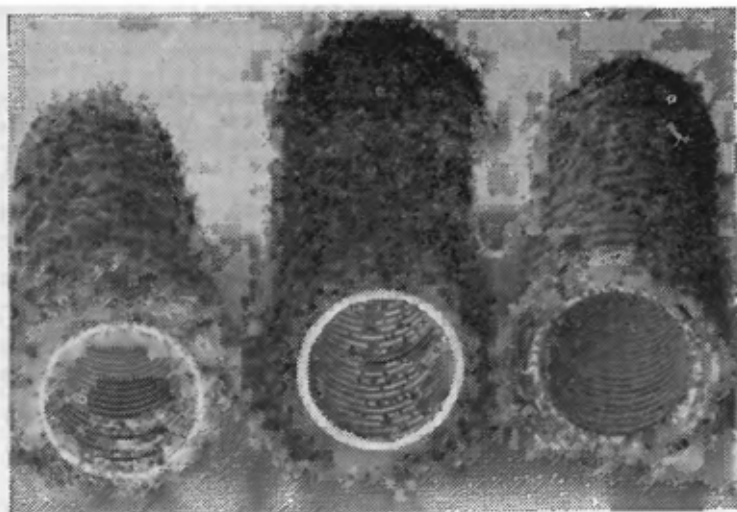
Рис. 8.16. Пластмассовые дренажные трубы, обернутые в фильтрующие материалы: слева направо — кокосовое волокно, полипропиленовое волокно и флутан из дуо (верхний слой) + торфяное волокно (внутренний слой).
