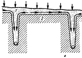
Рис. 5.5. Действие трубчатого дренажа в водопроницаемой почве [5.9]:
