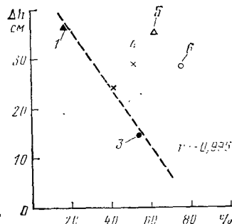
Рис. 5.19. Корреляция сопротивления на вход воды в дрена при свободных водовыпускных отверстиях дренажных труб из ПВХ [5.11]: 1 — без фильтра; 2 — солома; 3 — стружка; 4 — стекловолокно; 5 — филтан; 6 — дуб
