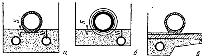
Рис. 7.16. Дренаж для осушения открытых котлованов и ,раншей канализации [7.14]: а — с двумя дренажными трубами без бетонного основания; б — с одной дренажной трубой без бетонного основания; в — с бетонным основанием.
