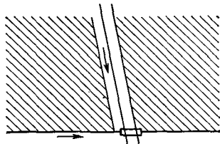
Рис. 7.6. Проведение всасывающих дрен при дорожном и другом строительстве.
