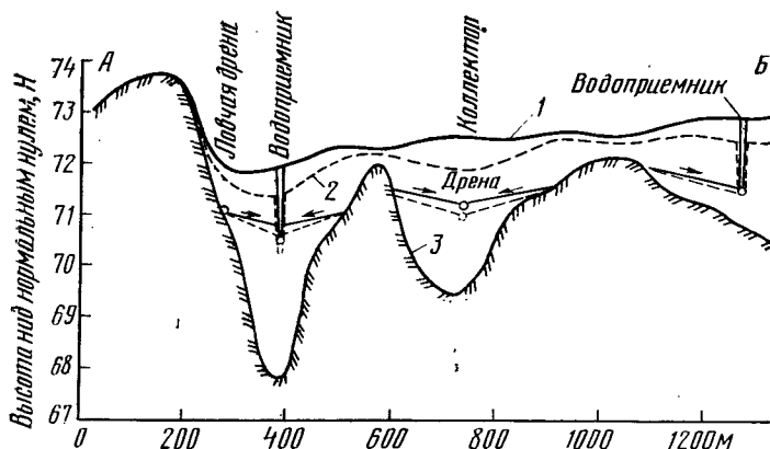
Рис. 3.3. Разрез местности по А—Б (см. рис. 3.2) до и после дренирования [3.2]:
