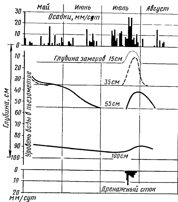
Рис. 5.16. Атмосферные осадки, верховодка и дренажный сток при комбинированном дренаже [4.7].
