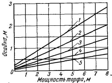
Рис. 7.10. Номограмма эмпирической формулы осадки торфа [7.25]:
