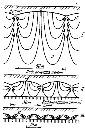
Рис. 5.4. Влияние глубины залегания водопроницаемого слоя почвы на расстояние между дренами:
