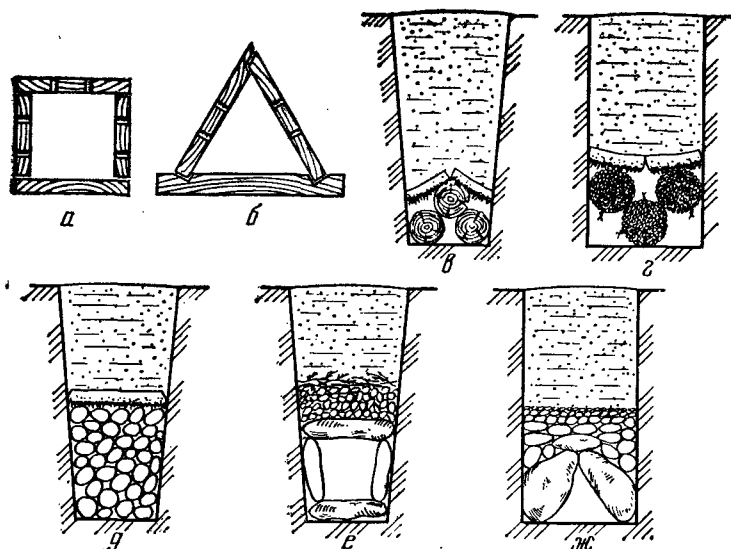
Рис. 9.16. Виды выполняемого вручную дренажа: а, б — деревянные дощатые дрены; в — жердевая дрена; г — фашинная дрена; д—ж — каменные дрены; в—г — дрены, покрытые дерниной.
