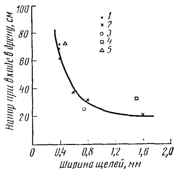
Рис. 5.14. Результаты измерения в полевых условиях сопротивления на вход в дренажи при разной ширине водонепроницаемых отверстий (щелей):
