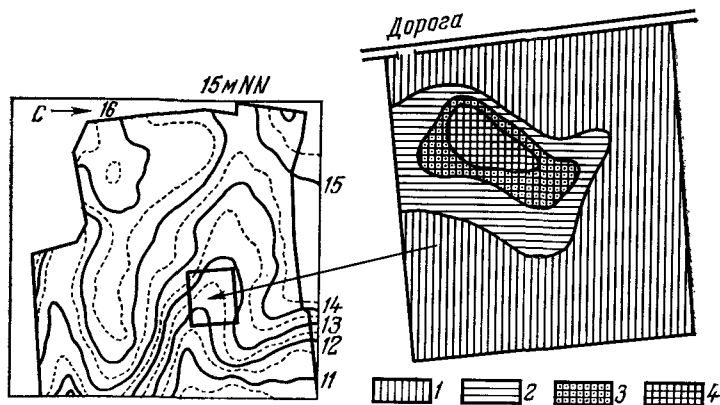
Рис. 3.18. Картирование растительности (вахта трехлистая Menianthes trifoliata ) и степень увлажнения почвы [3.4]:
