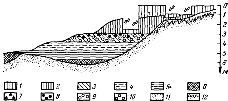
Рис. 2.9. Важнейшие профили болот в северной части ФРГ [3.2]: 1 — молодой мховый торф; 2 — старый мховый торф; 3 — торф разнороссы; 4 — осоковый торф; 5 — тростниковый торф; 6 — сфагнел; 7 — сосновые пни в торфе; 8 — сосновая древесина; 9 — березовая древесина; 10 — ольховая древесина; 11 — песок; 12 — орзанд.
