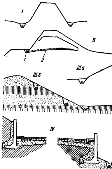
Рис. 7.15. Дренаж в подземном строительстве:
