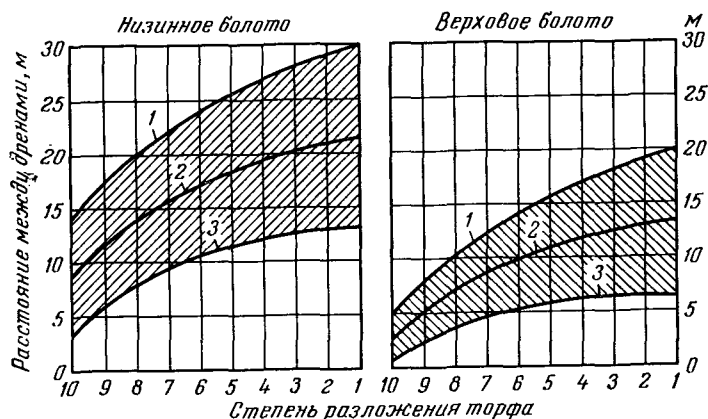
Рис. 7.12. Номограмма для определения расстояния между дренами на болотах северо-западной части ФРГ в зависимости от интенсивности предварительного осушения:
