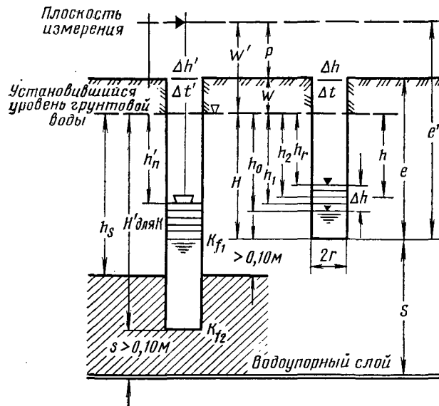
Рис. 3.12. Схема измерения водопроницаемости в буровой скважине [3.3].
