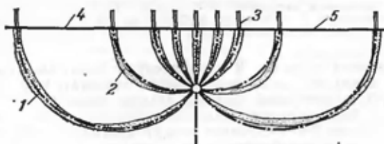
Рис. 5.2. Сравнение расчетных и окрашенных линий тока [5.14]:
