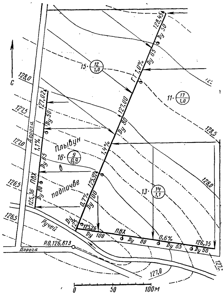
Рис. 7.22. План участка с трубчатым дренажем:
