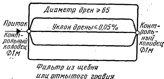
Рис. 7.19. Трубчатый дренаж для поверхностных самотечных поливов осветленными сточными водами, поступающими из жилых домов на одну—две семьи.
