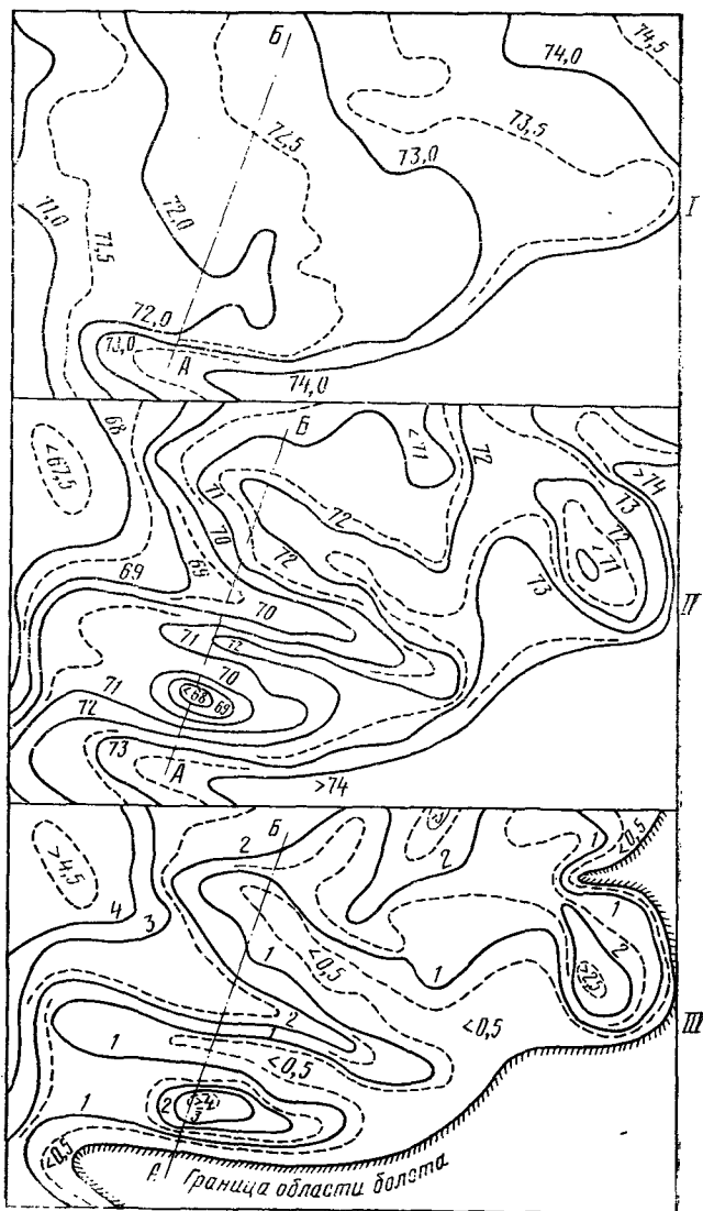
Рис. 3.2. План поверхности болота [3.2]. Разрез А—В на рисунках 3.3 и 3.7:
