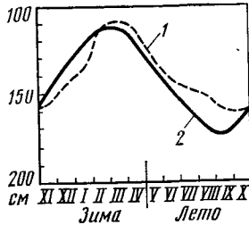
Рис. 2.5. Годовые колебания уровня грунтовых вод:
