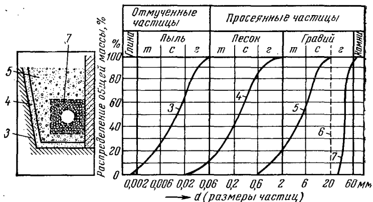
Рис. 7.14. Правила устройства фильтров Терцаги (стандарт ФРГ DIN 4095):
