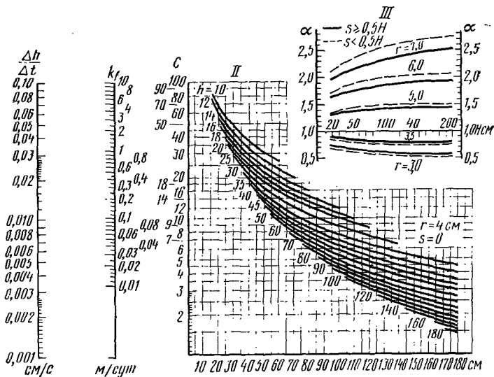
Рис. 3.13. Номограммы для определения в полевых условиях фильтрационной способности k_f при r=4 см [3.3]: I — для s \geq 0,5H ; II — для s < 0,5H ; III — для радиуса скважины r \neq 4 см.
