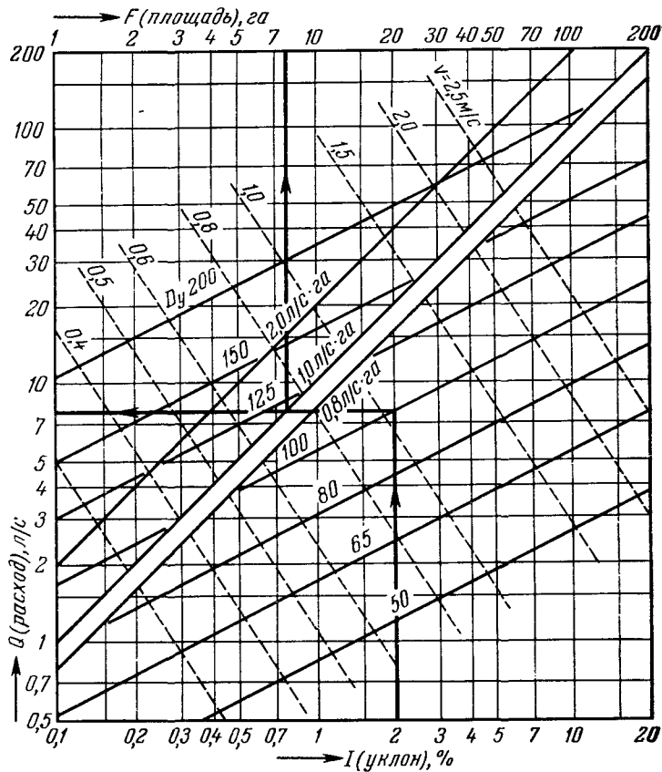
Рис. 6.1. Номограмма для определения внутреннего диаметра дрен, скорости воды и расходов. Дренажные трубы гошарные ( k_b=0,7 мм), D_y — внутренний диаметр.
