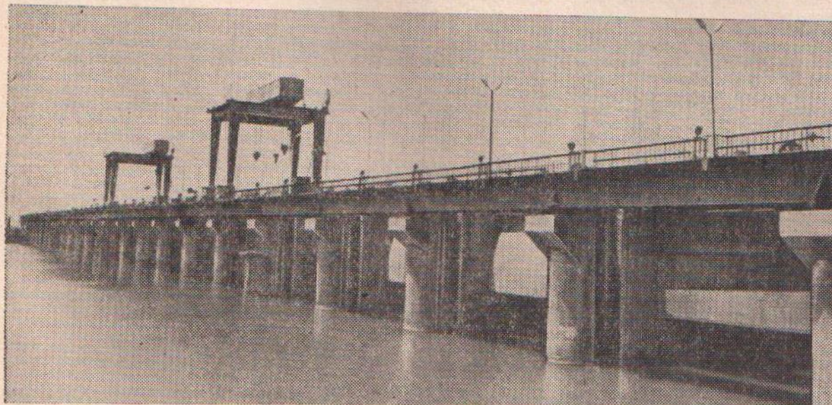
Каракалпакская АССР. На р. Амударье строится Тахиаташский гидроузел. Это крупное гидротехническое сооружение позволит улучшить условия судоходства и рыболовства, решит проблемы автомобильного и железнодорожного сообщения между левым и правым берегами Амударьи. С вводом его в действие улучшится водообеспеченность земель Ташаузской области Туркменской ССР и Каракалпакской АССР.
