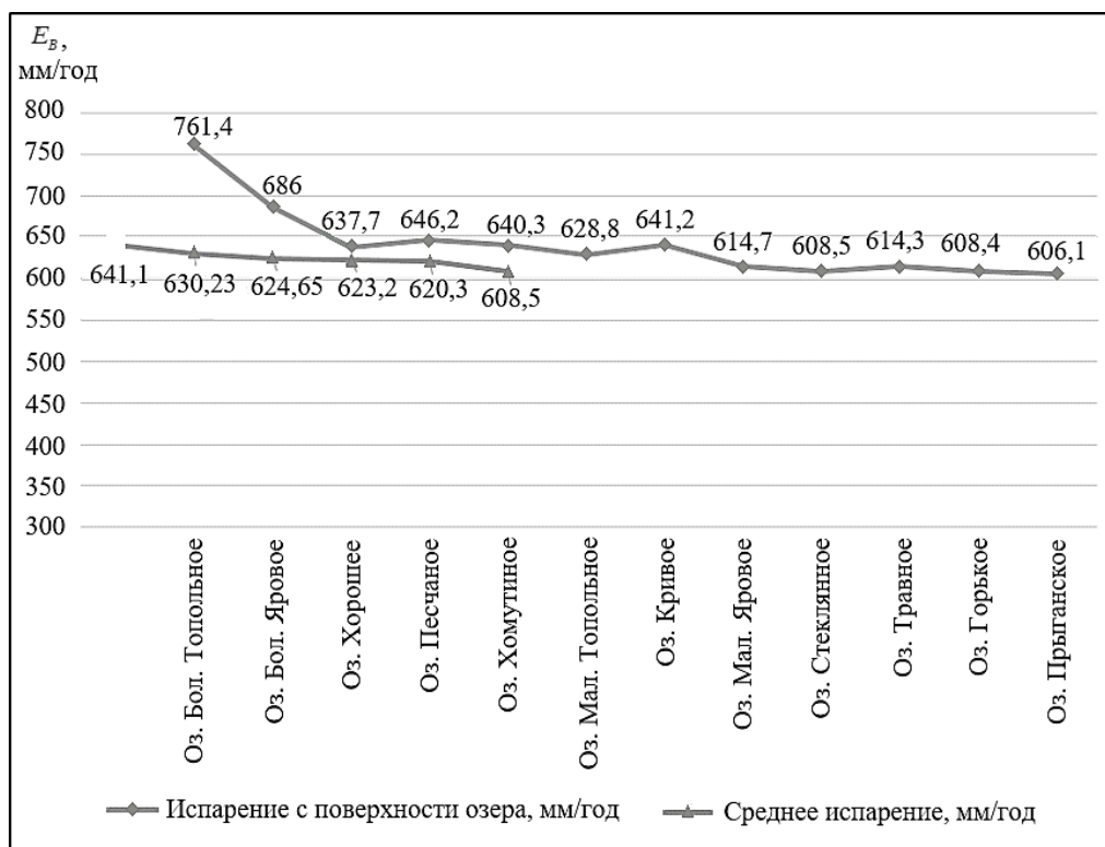
Рисунок 2 – График испарения с поверхности озер
