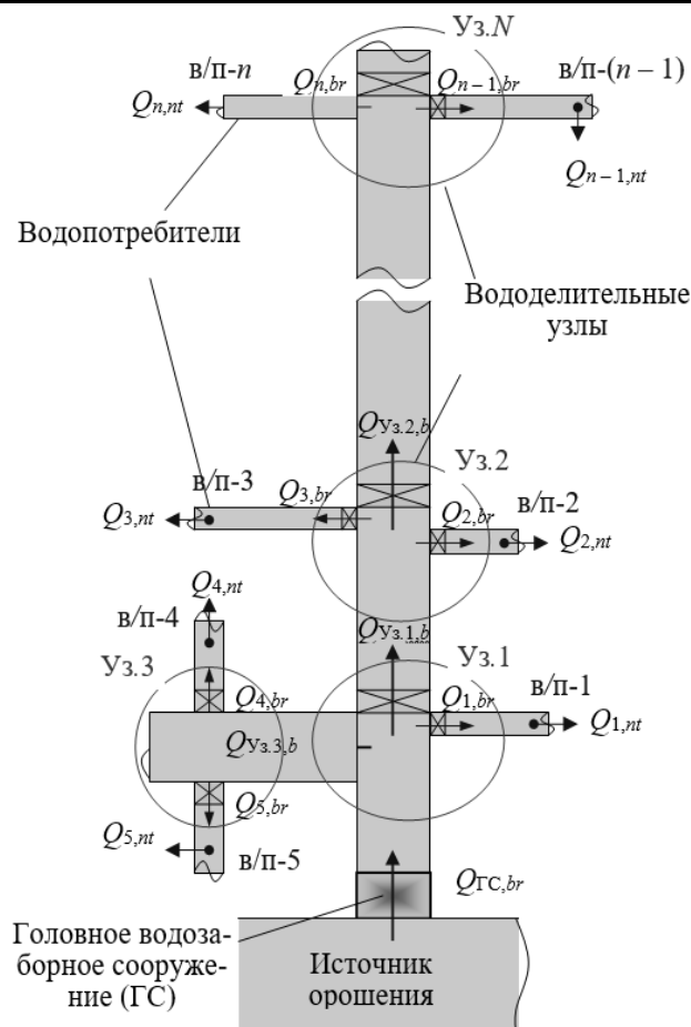
Рисунок 1 – Пример схемы водораспределительной сети, демонстрирующей процедуру построения алгоритма расчета
