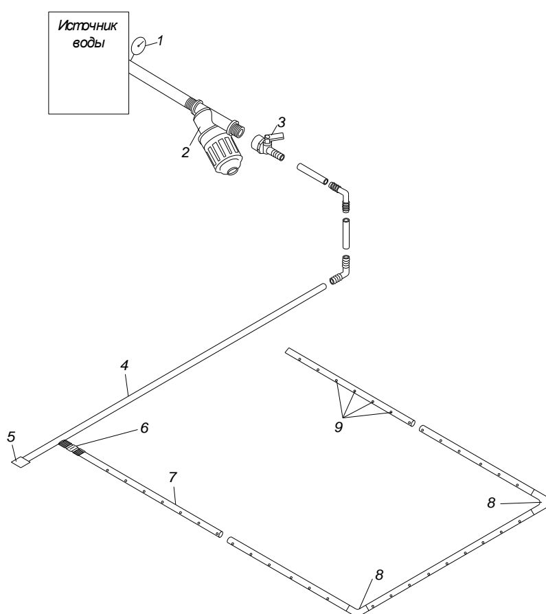
1 – манометр; 2 – фильтр; 3 – кран; 4 – транзитный трубопровод; 5 – заглушка; 6 – фитинг (кран); 7 – капельная лента (щелевая или эмиттерная); 8 – фитинг (отвод); 9 – капельницы
