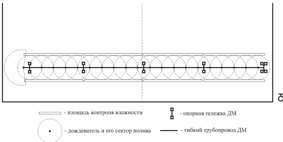
Рисунок 1 – Схема работы дождевальная машины фронтального действия, оснащенной гиперспектральной камерой, вид сверху
