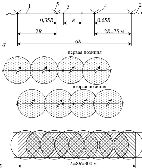
Рисунок 1 – Типовая схема размещения комплекта дождевального оборудования КИ-50
