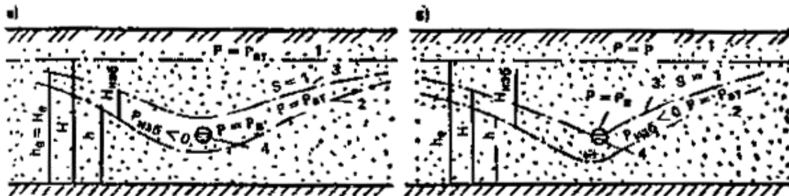
Рис. 99. Схемы к расчету фильтрации к горизонтальной дрене при вакуумировании на первом (а) и втором (б) этапах
