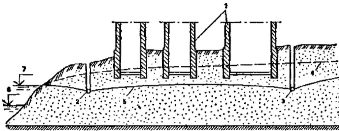
Рис. 57. Схема двухлинейного дренажа
