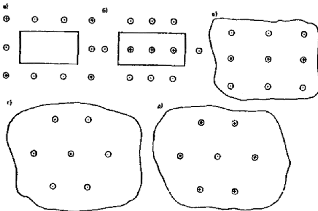
Рис. 56. Схемы планового расположения скважин пневмонагнетательных дренажей
