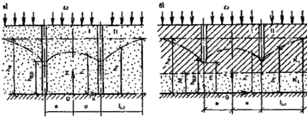
Рис. 73. Расчетные схемы двухлинейного дренажа
