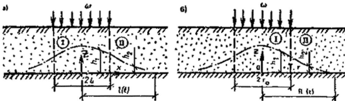
Рис. 2. Схемы к формированию техногенного водоносного горизонта на региональном водоупоре в первоначально сухих грунтах при поступлении инфильтрации из источника полосообразной (а) и круглой (б) в плане формы
