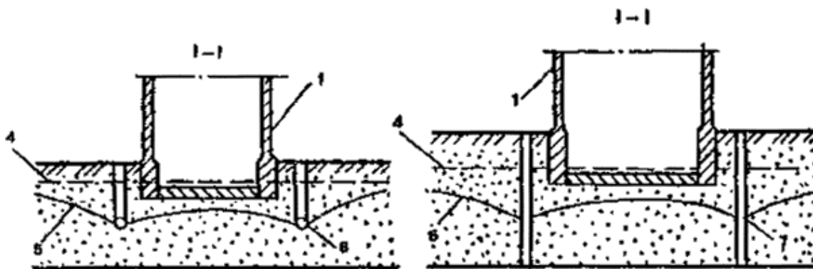
Рис. 59. Схема площадного дренажа
