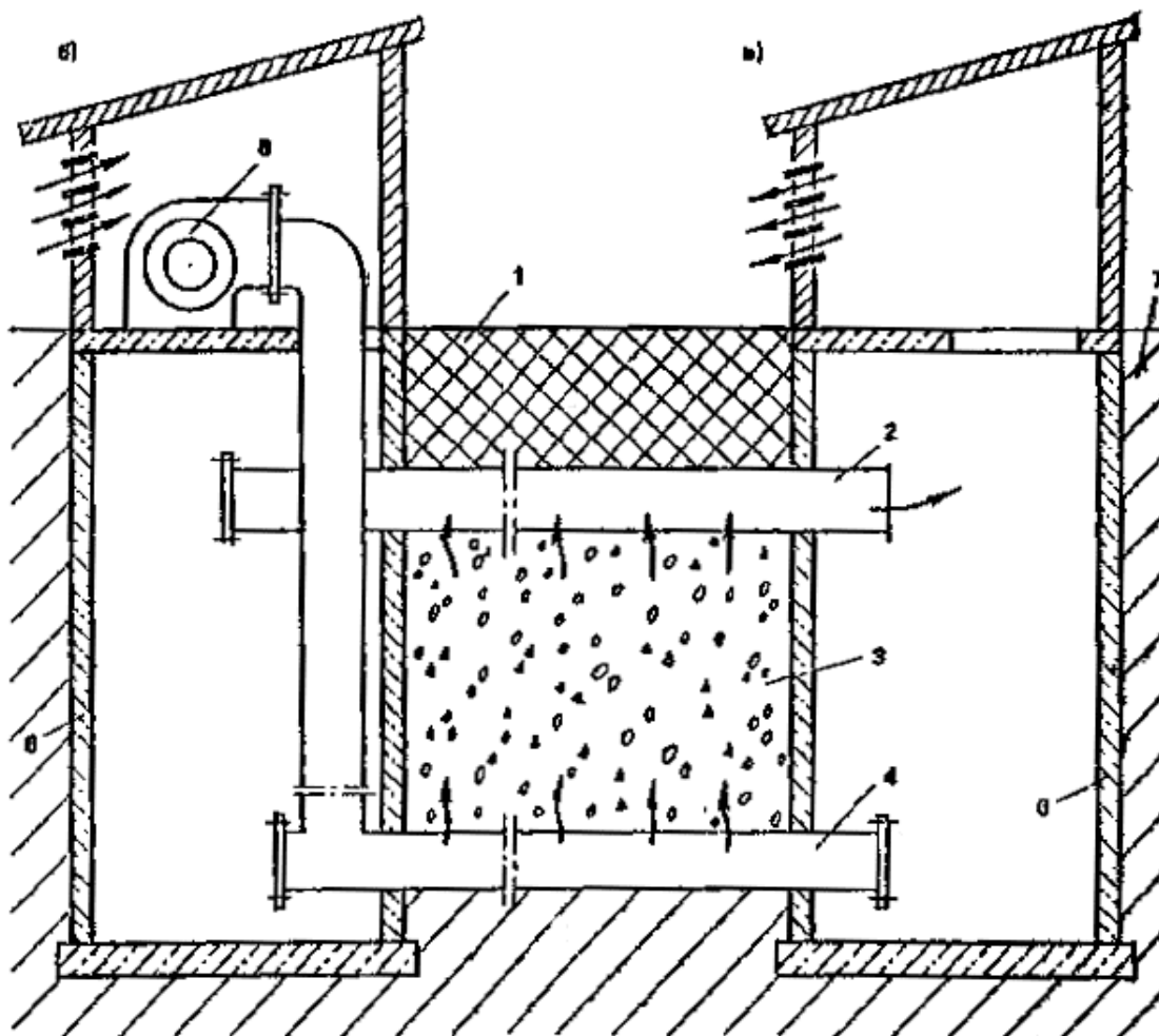
Рис. 31. Конструктивные схемы колодцев вентиляционного дренажа
