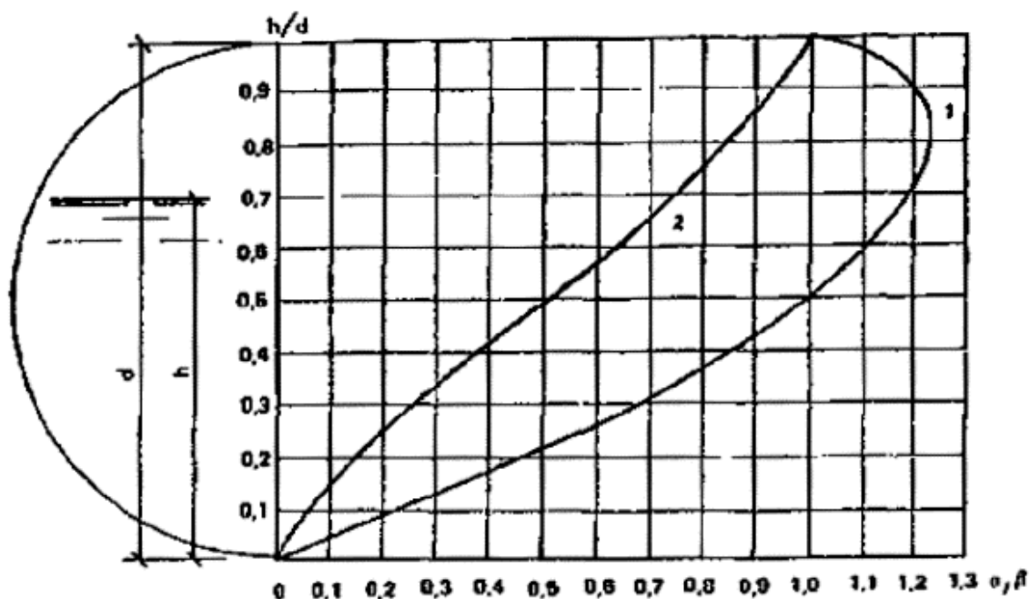
Рис. 132. Графики зависимости коэффициентов a и b от глубины наполнения ( h/d )
