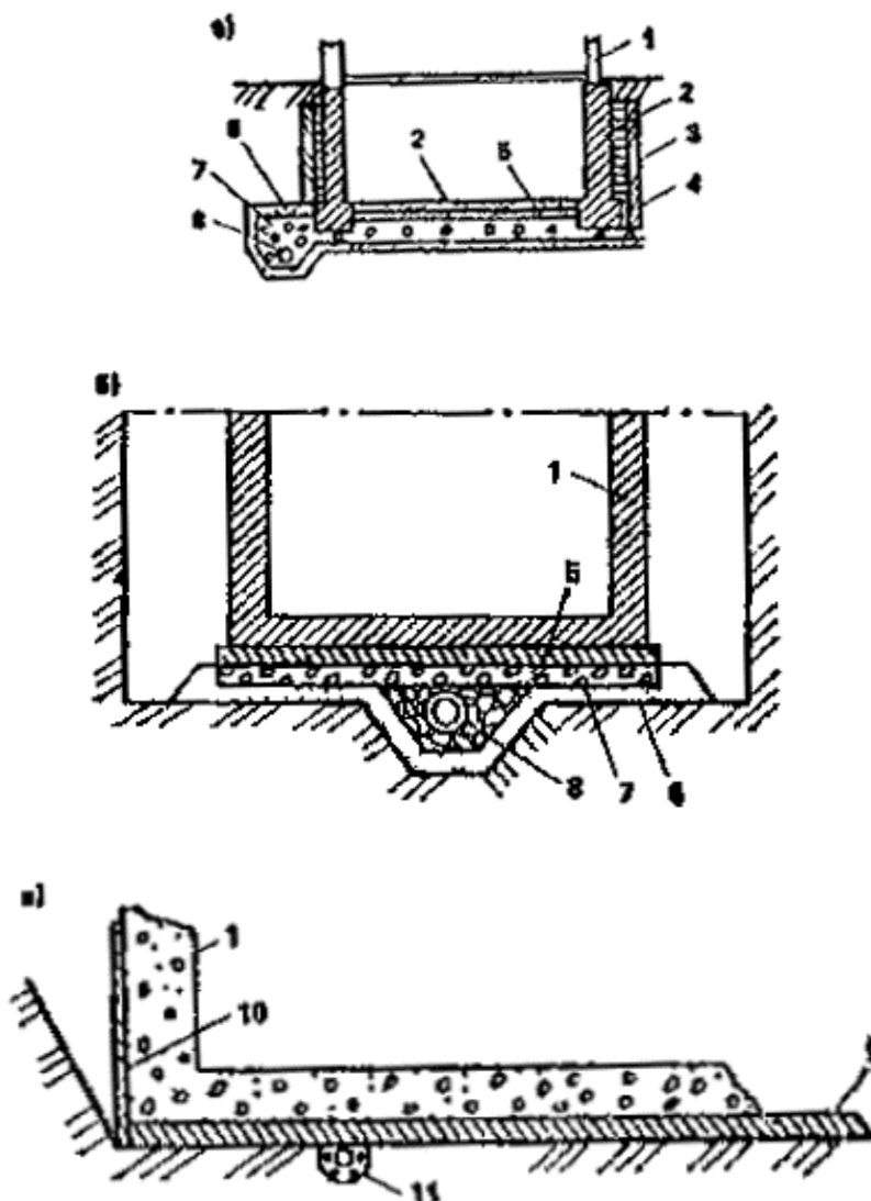
Рис. 27. Конструктивные схемы пластовых дренажей
