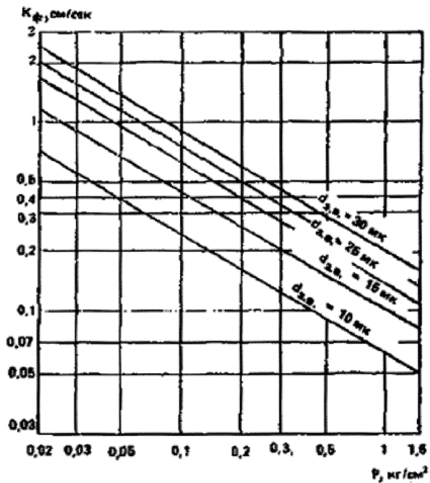
Рис. 130. График зависимости k_{\phi} = f(P, d_{\text{э.в}})
