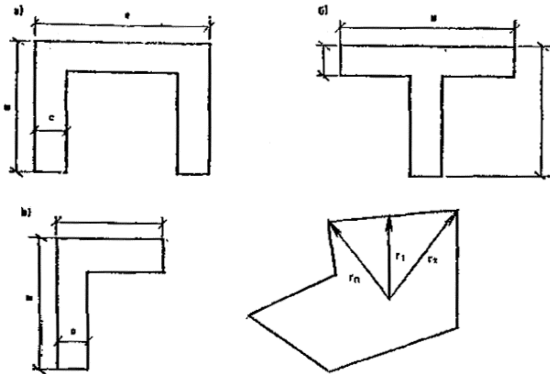
Рис. 76. Контурные дренажи различных в плане форм
