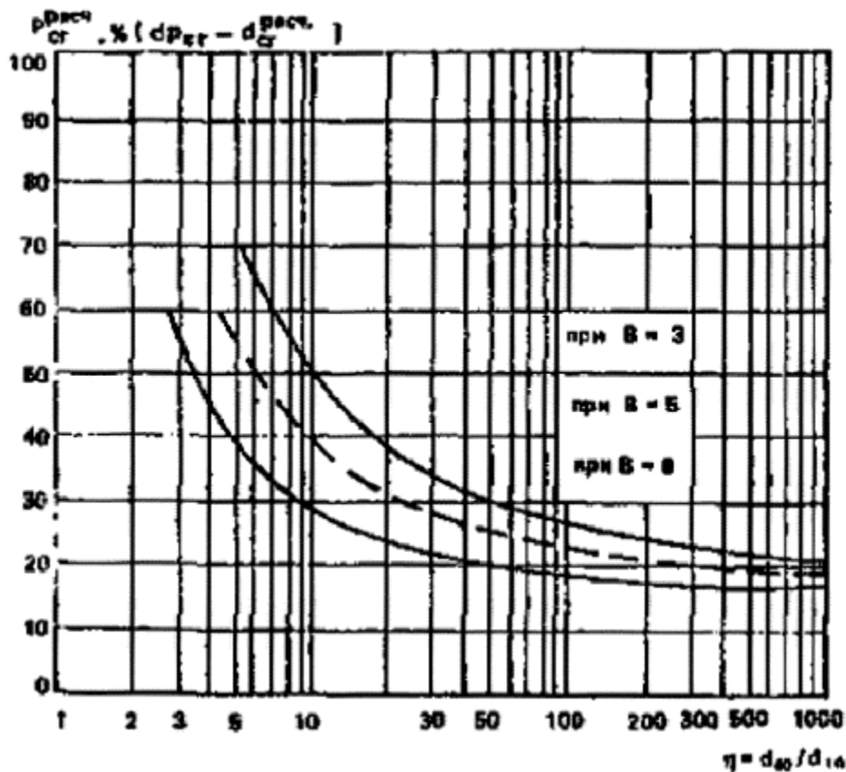
Рис. 124. График I_{\sigma}^{расч} = f(h_T) для определения расчетных размеров сводообразующих частиц грунта d_{сг}
