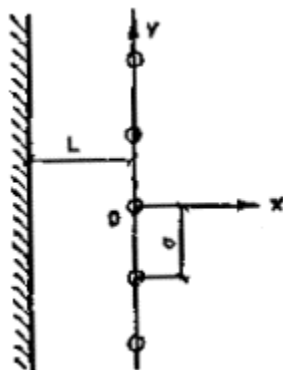
Рис. 114. Линейный ряд скважин в полуограниченном пласте
