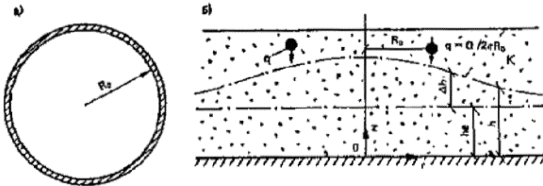
Рис. 16. Поступление дополнительной инфильтрации в пределах кольцевой зоны
