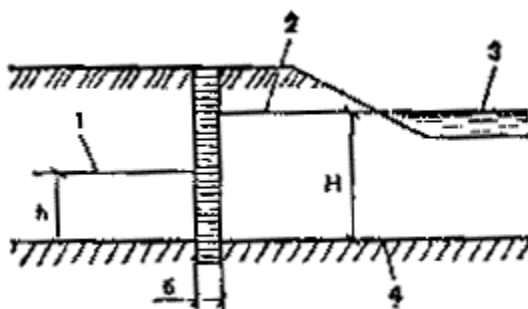
Рис. 32. Схема противофильтрационной завесы
