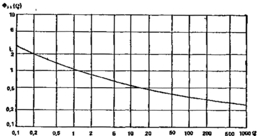
Рис. 88. График функции \Phi_{11}(f_0)
