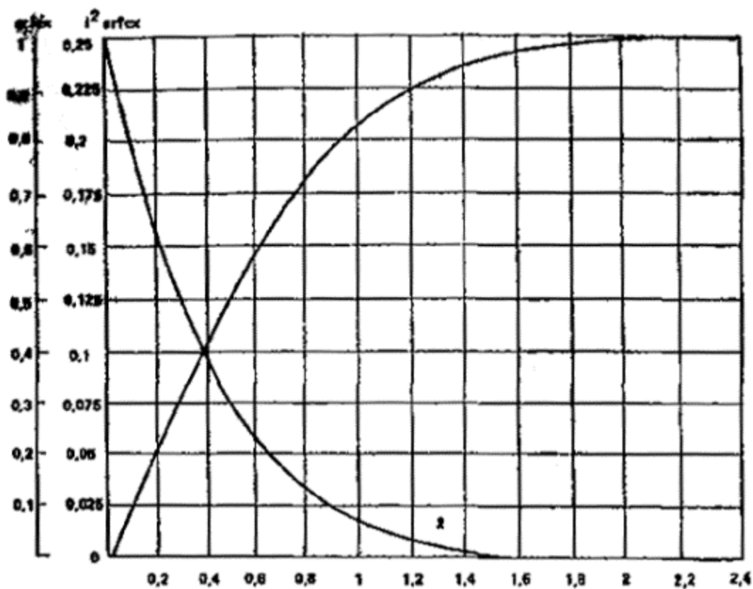
Рис. 3. График функций erf x (1) и i 2 erf x (2)
