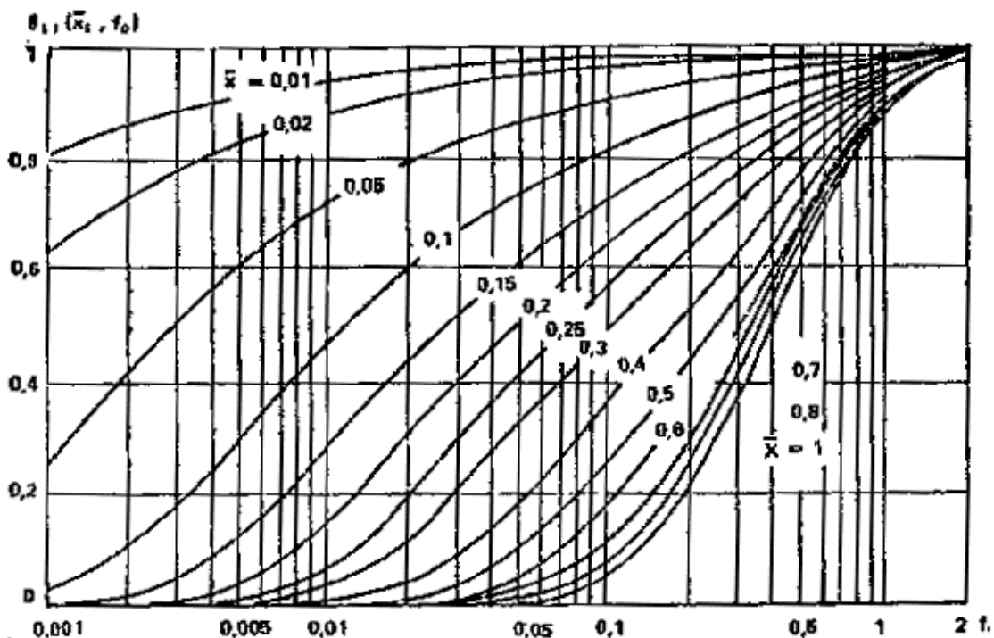
Рис. 102. График функции q_{11}(\bar{X}, f_0) .
