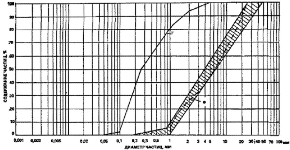
Рис. 135. Кривые гранулометрического состава к примеру подбора зернового состава фильтра для несвязанного несуггезионного грунта
