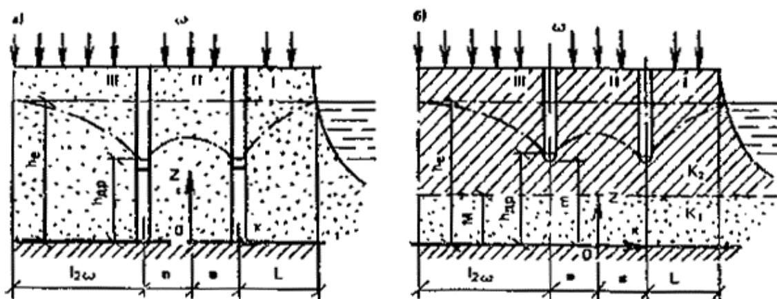
Рис. 75. Расчетные схемы двухлинейного берегового дренажа
