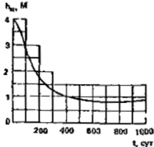
Рис. 119. График функции h (fo)
