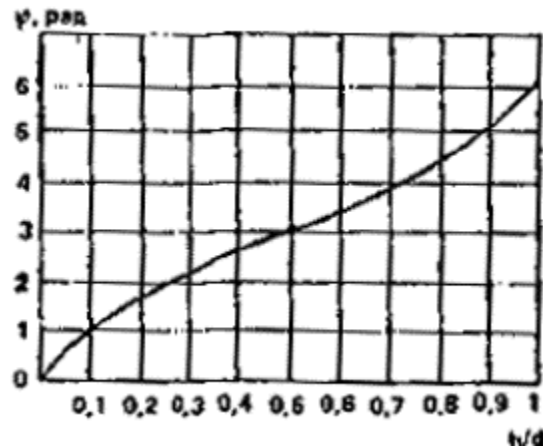
Рис. 123. График зависимости угла j от относительной глубины наполнения трубофильтра водой ( h/d )
