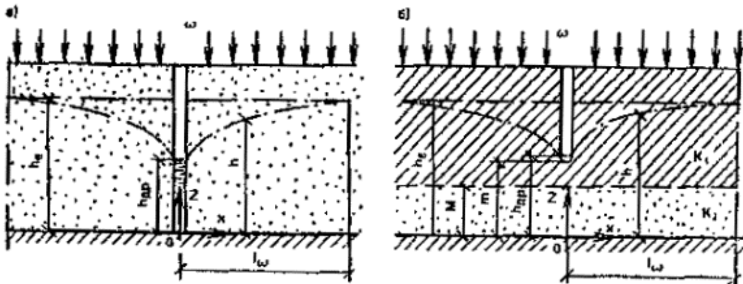
Рис. 72. Расчетные схемы однолинейного дренажа
