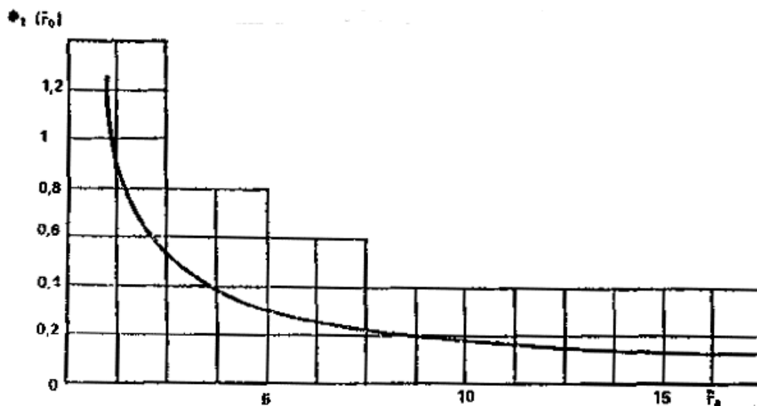
Рис. 83. График функции F_7 (\bar{r}_0)
