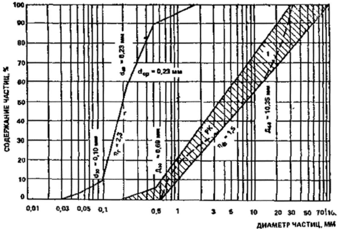
Рис. 126. График запроектированного состава фильтра
