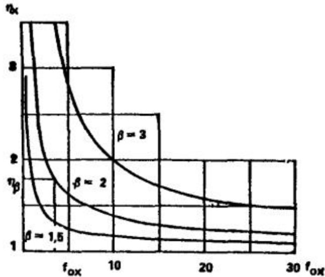
Рис. 23. График зависимости h_x от f_{0x}
