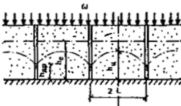
Рис. 63. Схема к определению безопасного расстояния от защищаемого сооружения до дренажа
