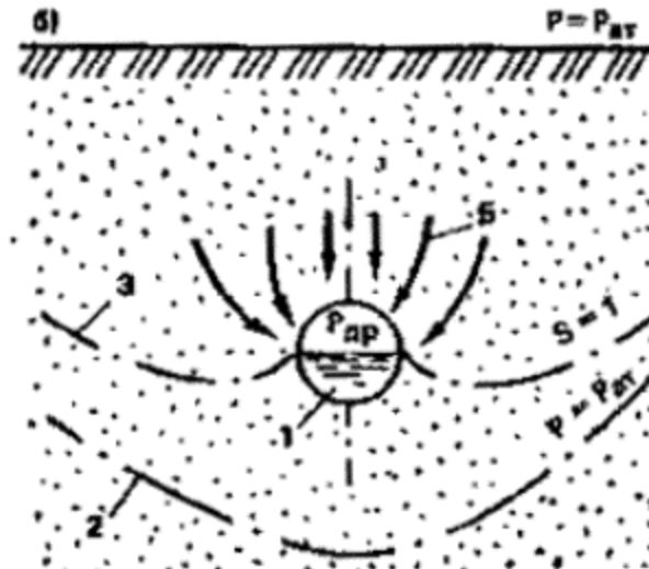
Рис. 103. Схемы к расчету притока воздуха в вакуумный дренаж после его прорыва при наличии (а) и отсутствии (б) защитного экрана
