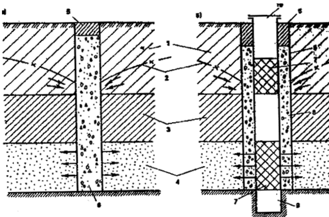
Рис. 47. Схемы конструкций вертикальных поглощающих дренажных скважин
