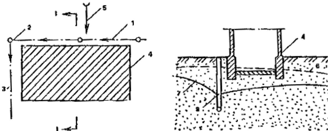
Рис. 35. Схема головного дренажа
