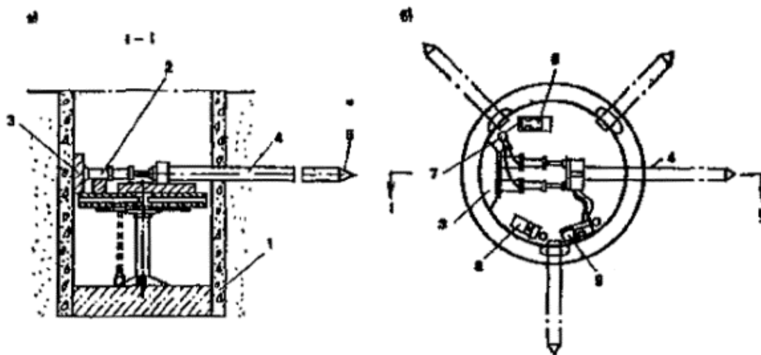
Рис. 44. Схема проходки лучевого дренажа
