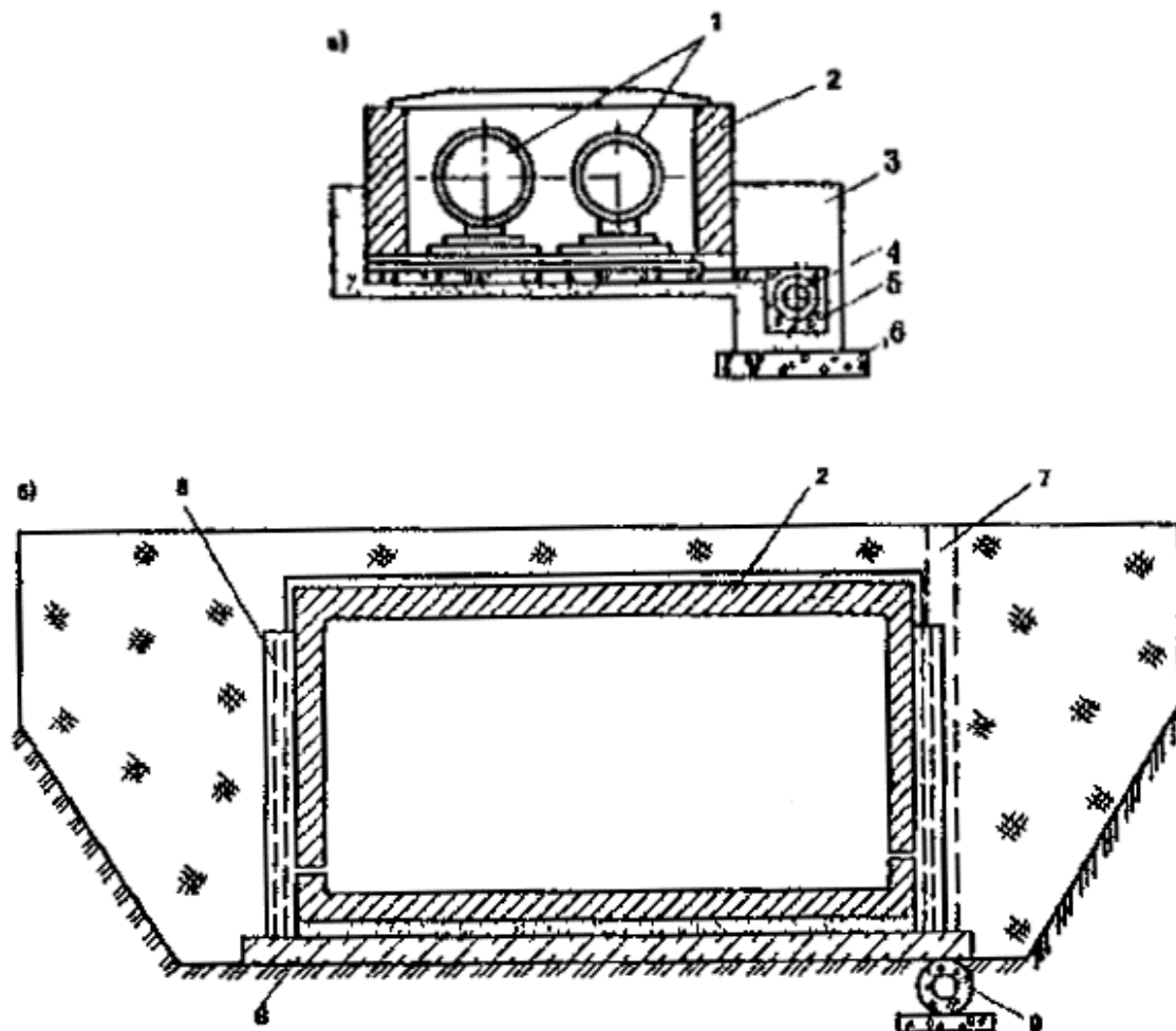
Рис. 28. Конструктивные схемы пластовых сопутствующих дренажей
