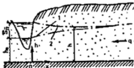
Рис. 18. Подпор грунтовых вод в полубесконечном массиве
