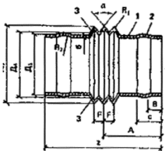
Рис. 40. Конструкция гибкой соединительной муфты
