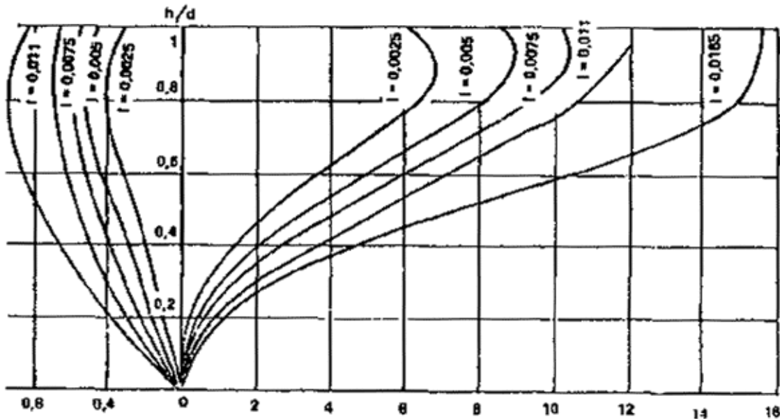
Рис. 134. График для гидравлического расчета горизонтального дренажа из трубофильтров диаметром 150 мм
