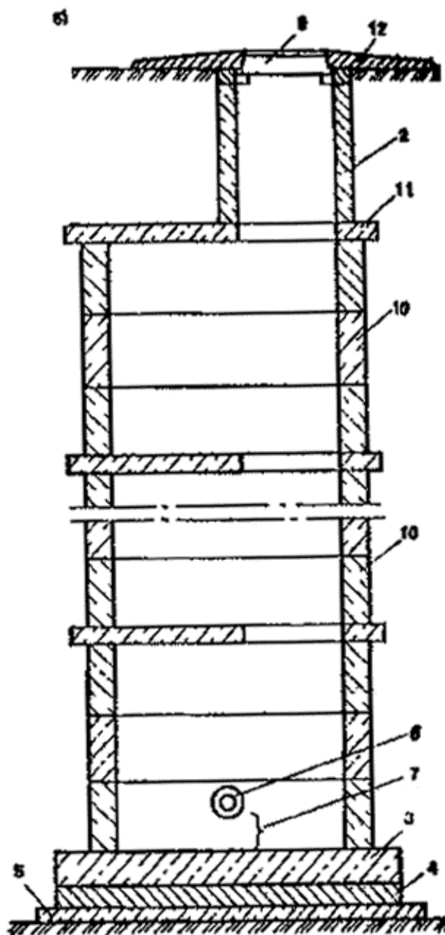
Рис. 60. Схема конструкции смотрового дренажного колодца
