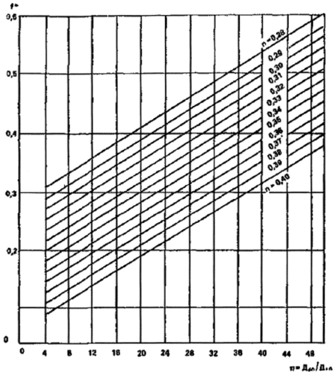
Рис. 127. График f^* = f(h)
