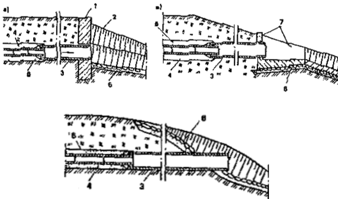
Рис. 62. Конструктивные схемы устьевых выпусков дренажных вод
