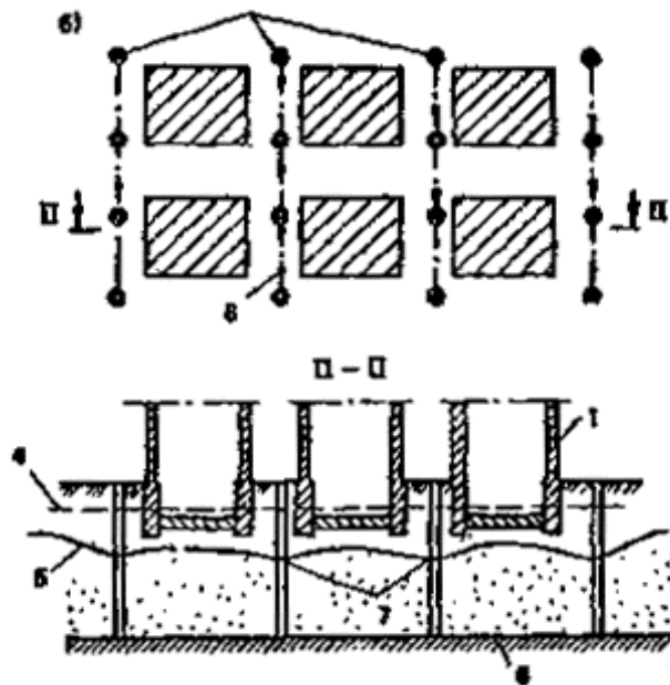
Рис. 58. Схема кольцевого дренажа
