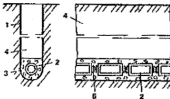
Рис. 41. Конструкция дрена с применением гибких соединительных муфт
