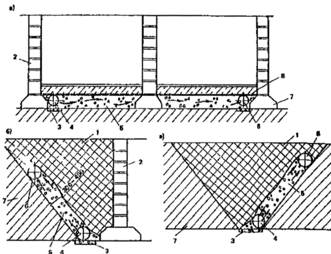
Рис. 29. Типы вентиляционного дренажа
