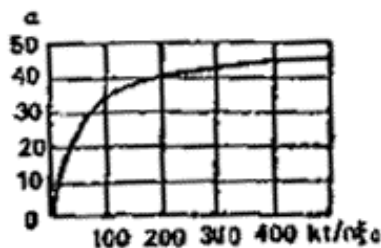
Рис. 24. Зависимость a от kt/(n\chi_0)
