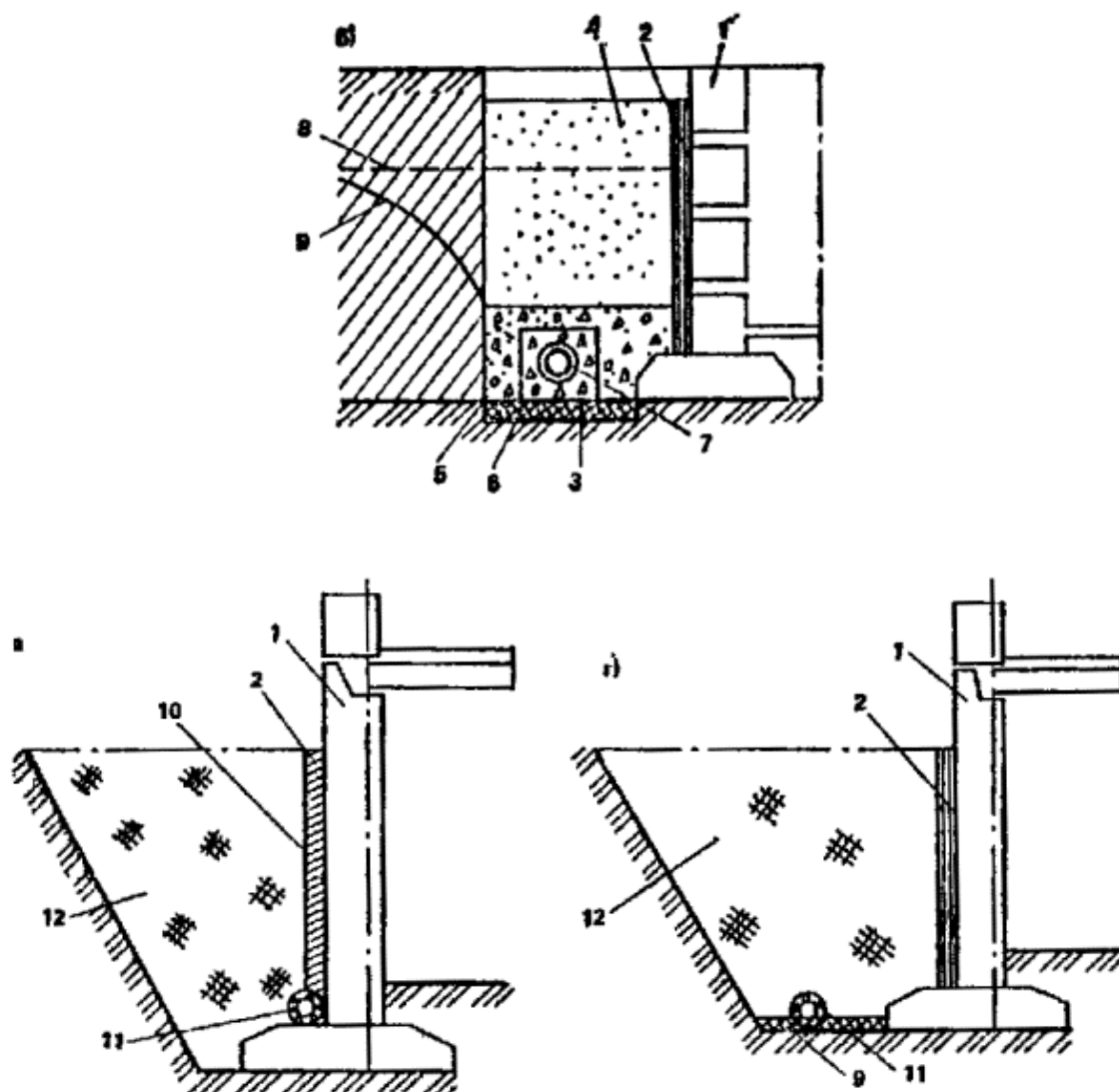
Рис. 26. Конструктивные схемы пристенных дренажей
