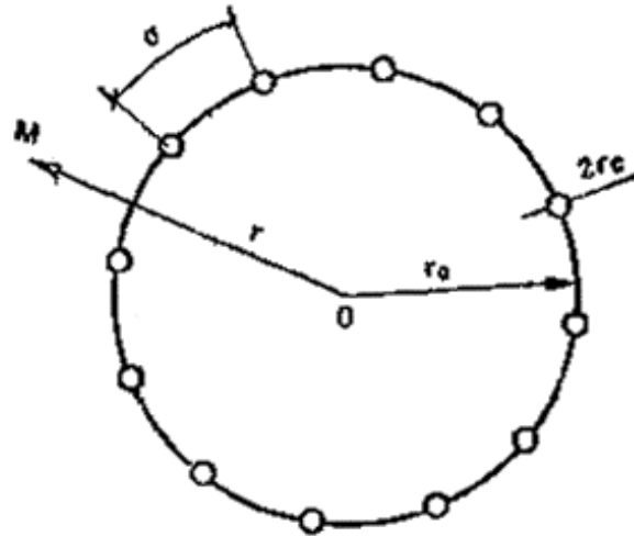
Рис. 115. Кольцевая система скважин в неограниченном пласте
