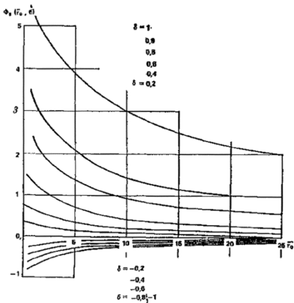
Рис. 85. График функции \Phi_8 (
