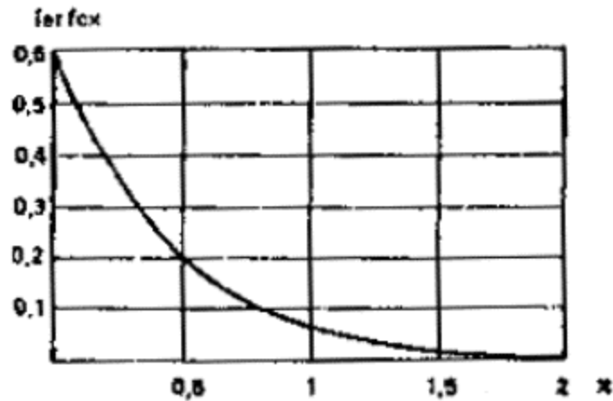
Рис. 11. График функции ierfc\ x .
