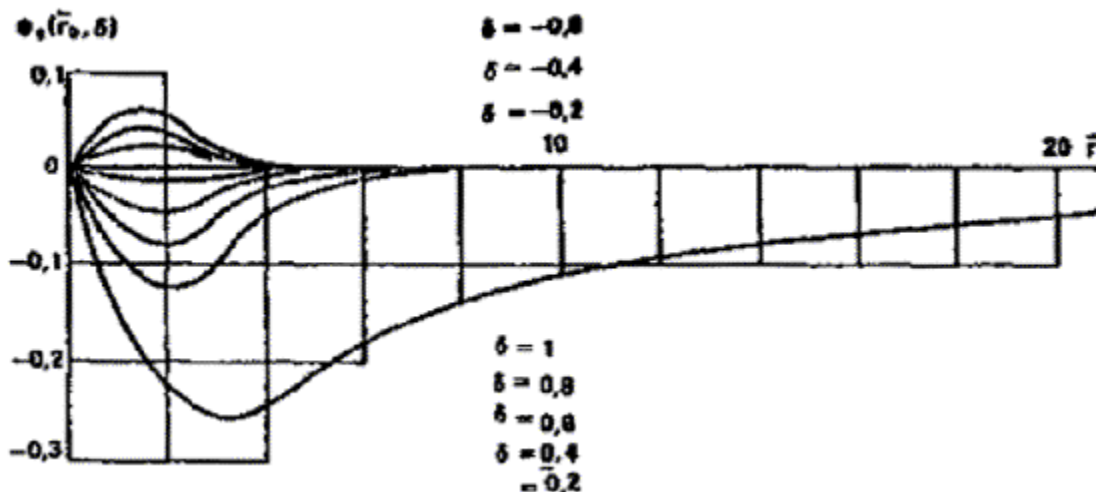
Рис. 86. График функции \Phi_9 (
