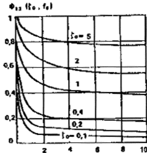
Рис. 93. График функции \Phi_{15}(\zeta_0, f_0)
