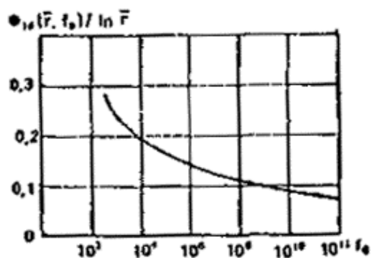
Рис. 118. График функции \Phi_{16}(\bar{r}, f_0)
