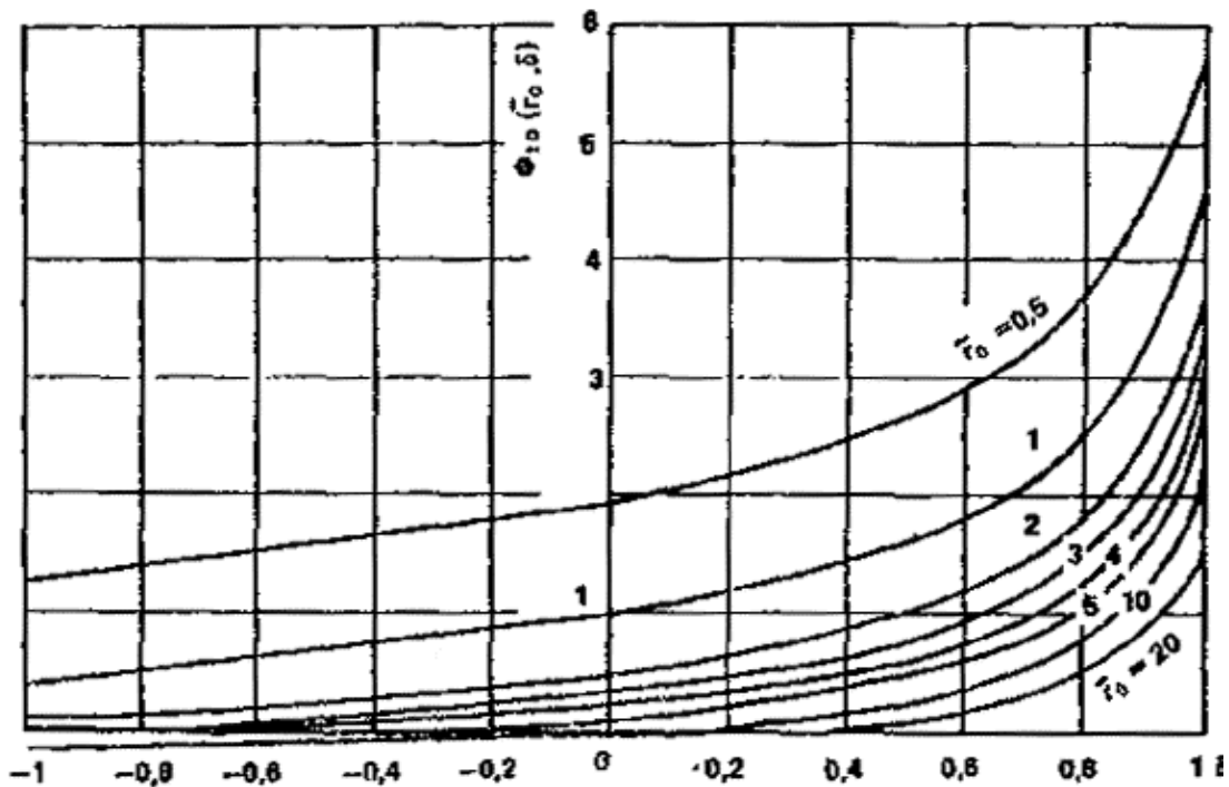
Рис. 87. График функции \Phi_{10} (
