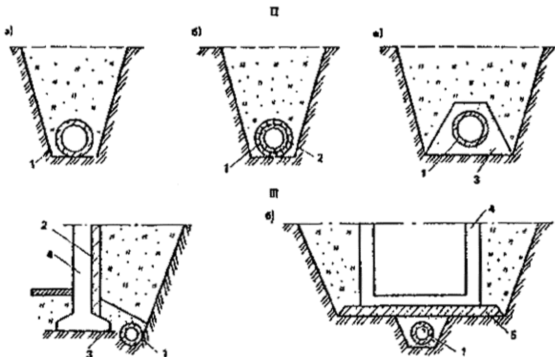
Рис. 39. Конструкции дренажей с применением трубофильтров
