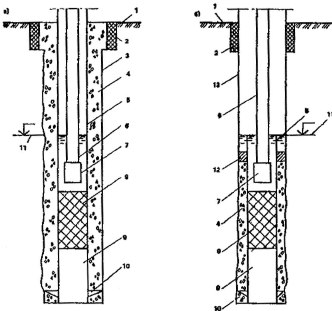
Рис. 46. Схемы конструкций скважин вертикального дренажа
