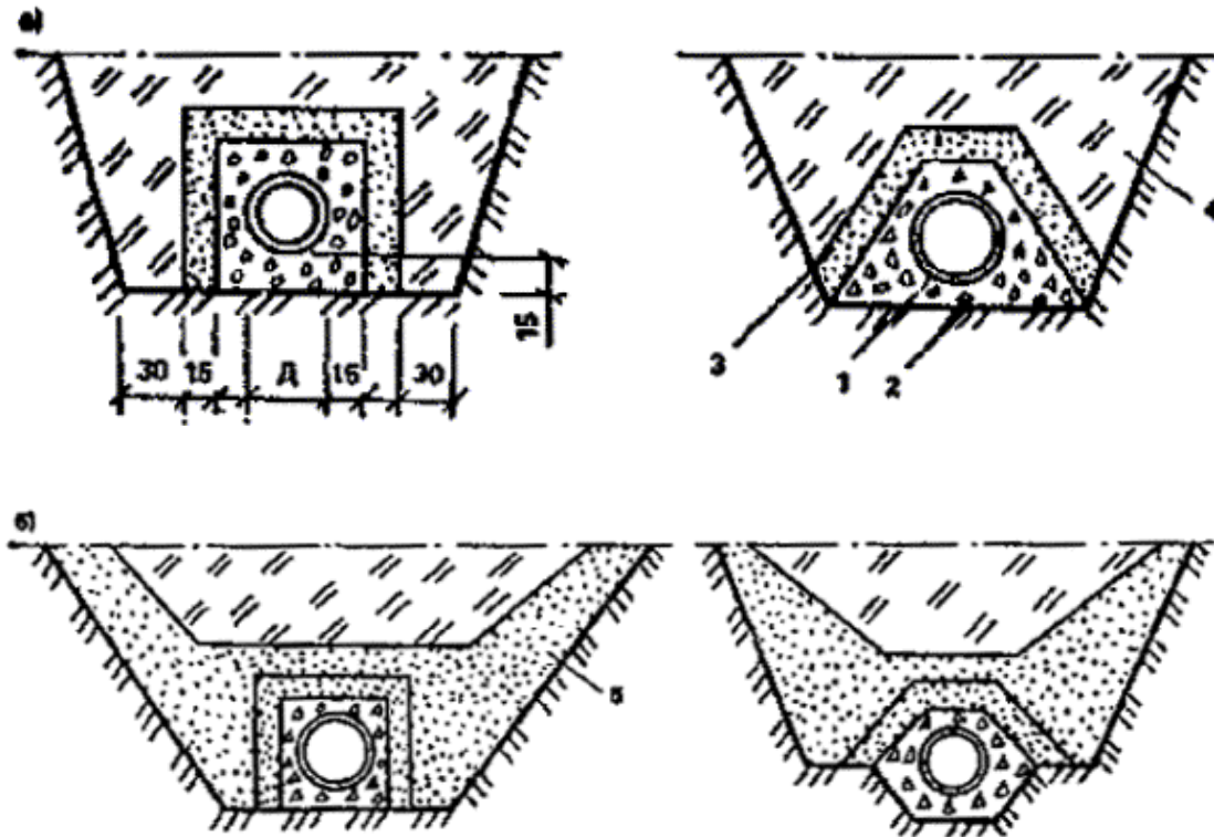
Рис. 37. Конструктивные схемы горизонтальных трубчатых дренажей, укладываемых в траншею
