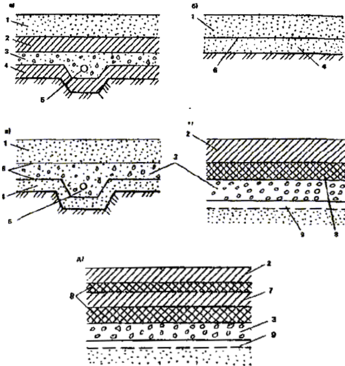
Рис. 34. Схемы противодиффузионных экранов
