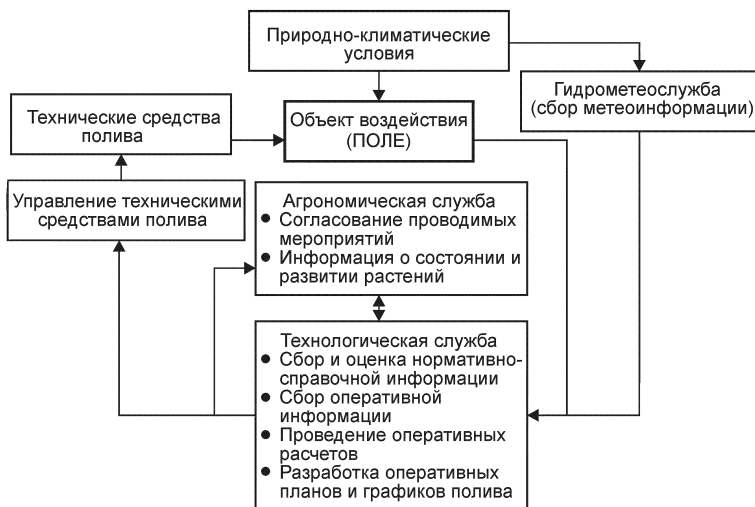
Рис. 15. Структурно-функциональная схема оперативного управления поливами
