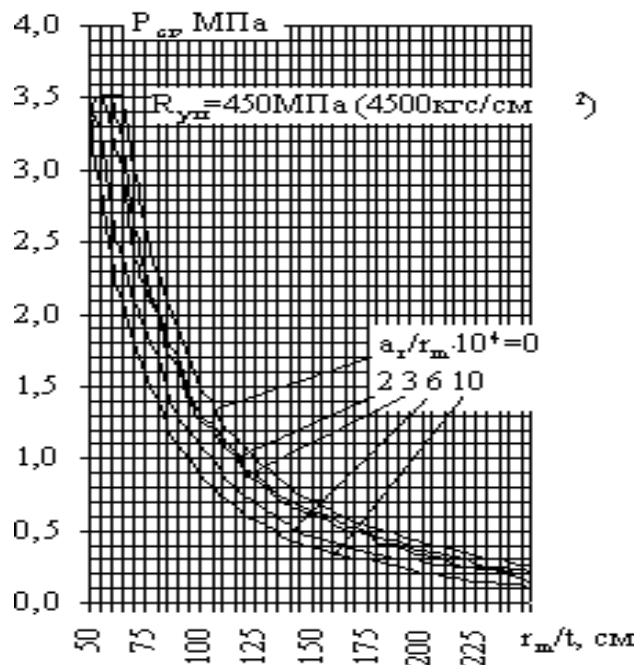
Черт. 2. График зависимости критического наружного давления P_{cr} от относительной толщины стенки r_m/t [ R_{yn} - нормативное сопротивление по пределу текучести стали, МПа ( \text{кгс/см}^2 );
