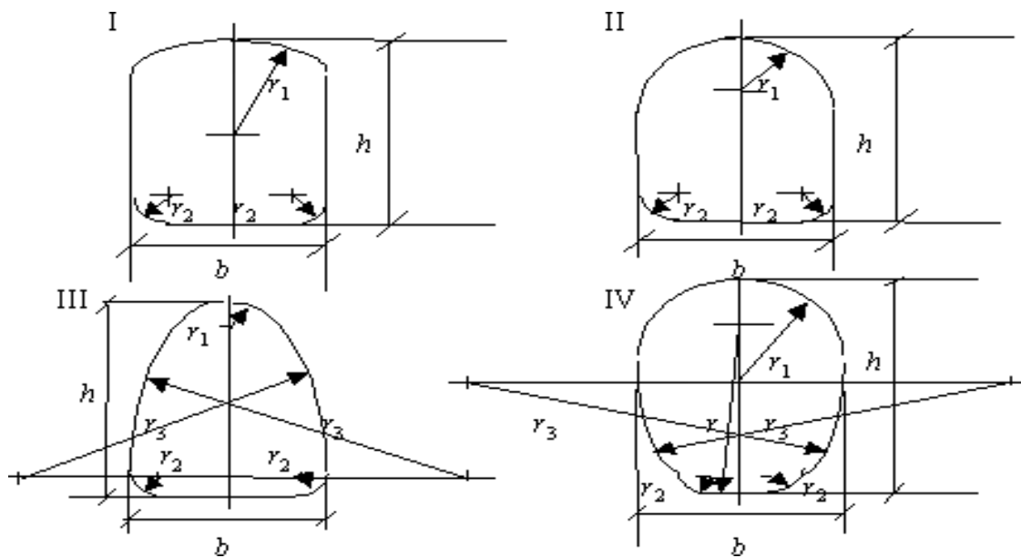
Черт. 1. Формы поперечных сечений безнапорных туннелей в свету
