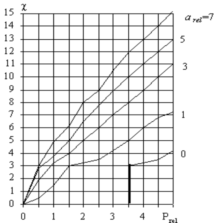
Черт. 3. График зависимости коэффициента c от p_{rel} при a_{rel} = \text{const}
