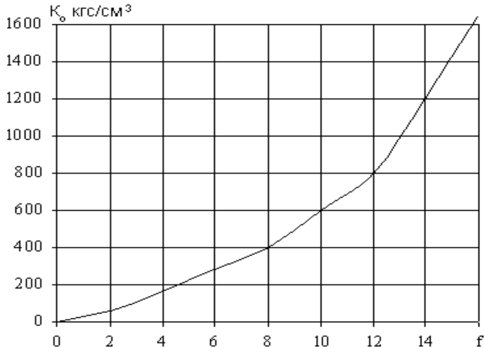
Черт. 2. График зависимости коэффициента K_0 от коэффициента крепости грунта f для трещиноватых грунтов
