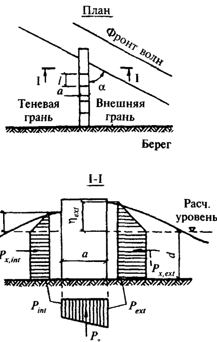
Рис. 30. Эпюры волнового давления на буню
