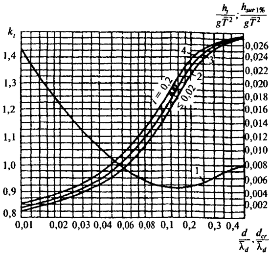
Рис. 5. Графики для определения 1 — коэффициента k_r ; 2, 3 и 4 — величин d_{cr}/\bar{\lambda}_d
