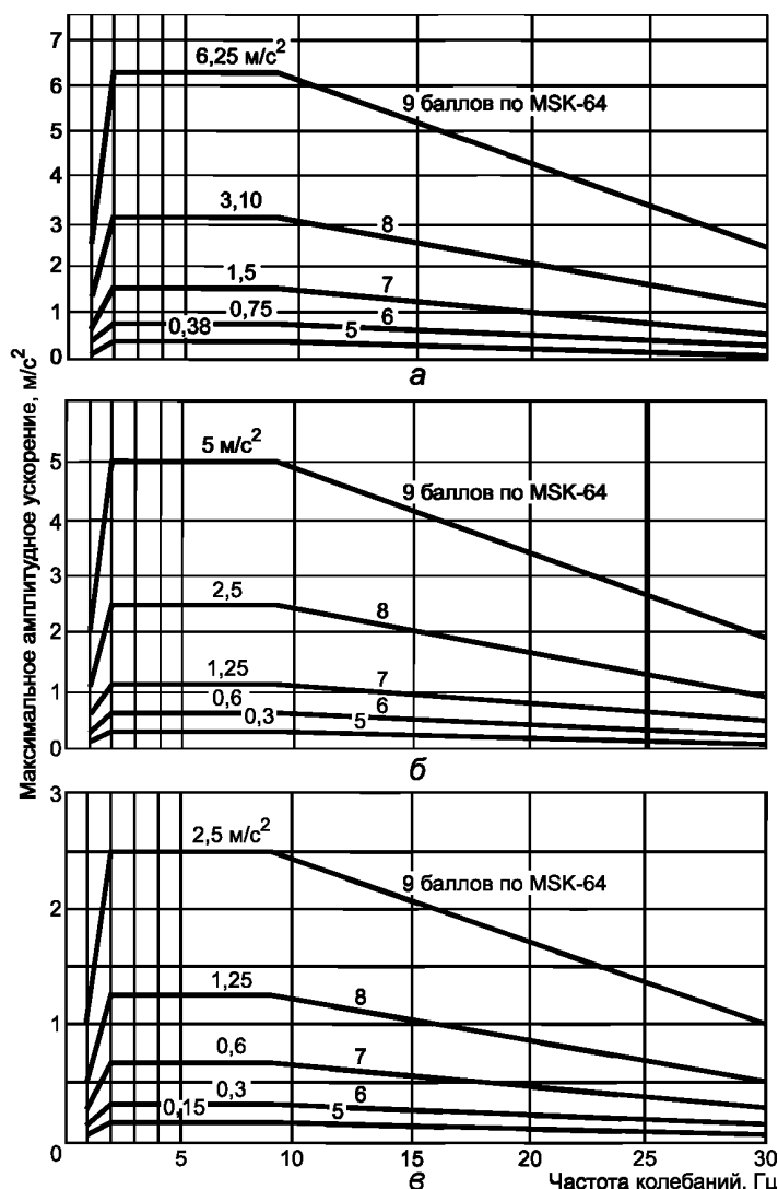
а — при высоте установки оборудования над нулевой отметкой 70—30 м; б — при высоте установки оборудования над нулевой отметкой 25 м; в — при высоте установки оборудования над нулевой отметкой 0—10 м
